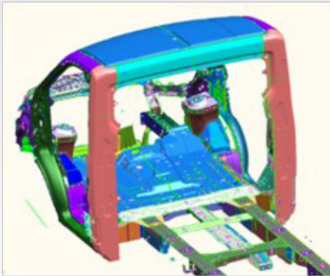
CAD-kuva: Takapaneeli poistettu
